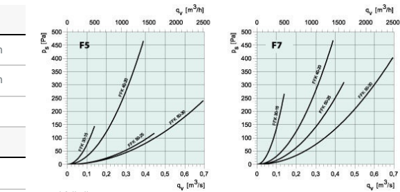
Tryckfallsdiagram
