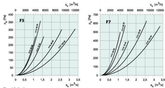
Tryckfallsdiagram
